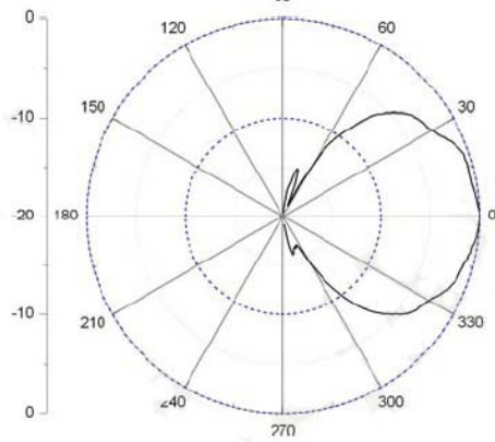
H-Plane
