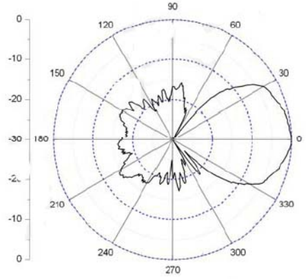
E-Plane
